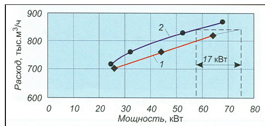
Рис. 11. Результаты испытаний вентиляторов АВО типа 1АВ3 на КС «Кушэвская» ООО «Кубаньгазпром»: 1 – Т-50-6; 2 – ГАЦ-50-6М2
