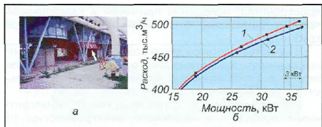
Рис. 6. Влияние установки коллектора плавного входа на характеристику вентилятора ГАЦ-50-4М2 (КС «Курская» ООО «Мострансгаз»): а - внешний вид коллектора (показан стрелкой); б - характеристики вентилятора с коллектором (1) и без него (2)
