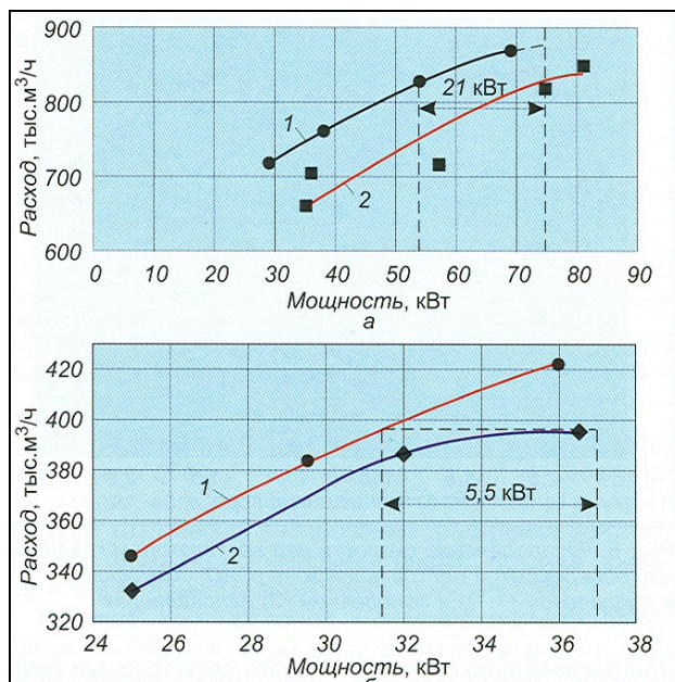
Рис. 7. Влияние центрального тела на характеристику вентилятора ГАЦ-50-6М2 АВО типа 1АВ3 КС «Кушэвская» ООО «Кубаньгазпром» (а); вентилятора ГАЦ-50-4М3 АВО типа 2АВГ-75 КС «Курская» ООО «Мострансгаз» (б): 1 - с центральным телом; 2 - без него
