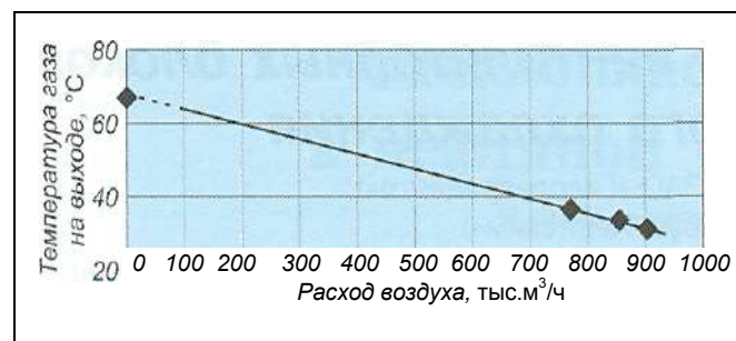
Рис. 2. Сравнение данных испытаний (♦) на КС «Курская» ООО «Мострансгаз» с результатом расчета (---) при расходе газа 357 тыс. м 3 /ч и температуре воздуха на входе 13°C
