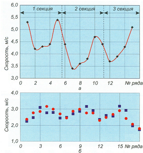
Рис. 4. Распределение скорости воздушного потока: а - АВО типа 2АВГ-75 КС «Курская» ООО «Моострансгаз»; б - АВО типа АВЗД КС «Октябрьская» ООО «Моострансгаз»; ■ - без уплотнения; • - с уплотнениями
