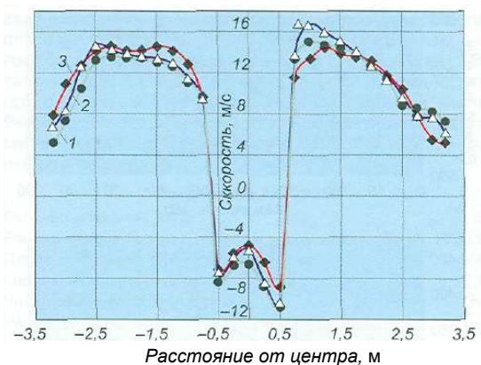
Рис. 5. Распределение скорости над вентилятором градирни при неперекрываемой центральной зоне (ОАО «Аммофос») в продольном (1, 2) и поперечном (3) направлениях
